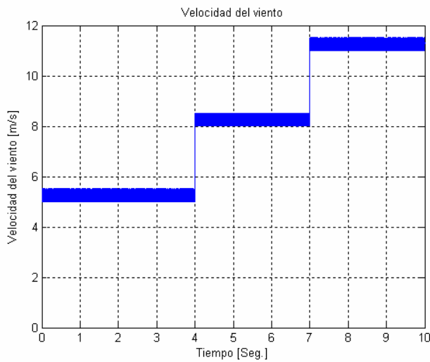
Figura 5.1: Velocidad del viento empleada para observar el desempeño del sistema. La señal presenta variaciones aleatorias sobre tres diferentes niveles de velocidad del viento en forma escalonada.
