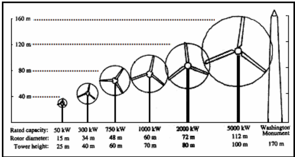
Figura 2.9 Capacidades y dimensiones principales de las turbinas de viento usadas en la actualidad [14].
