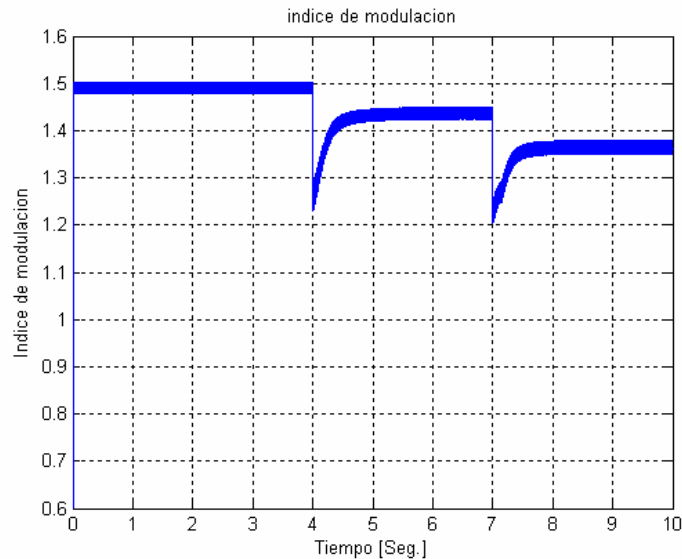
Figura 5.10: Comportamiento del índice de modulación ante variaciones mecánicas en la energía del primer motor.
