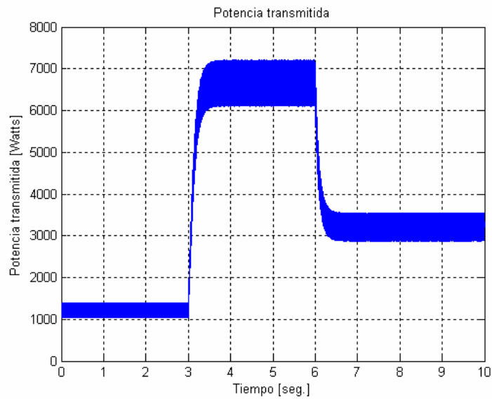
Figura 5.25: Potencia transmitida a la red en respuesta a las variaciones mecánicas en la energía del primer motor.
