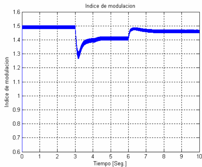
Figura 5.26: Comportamiento del índice de modulación ante variaciones mecánicas en la energía del primer motor.
