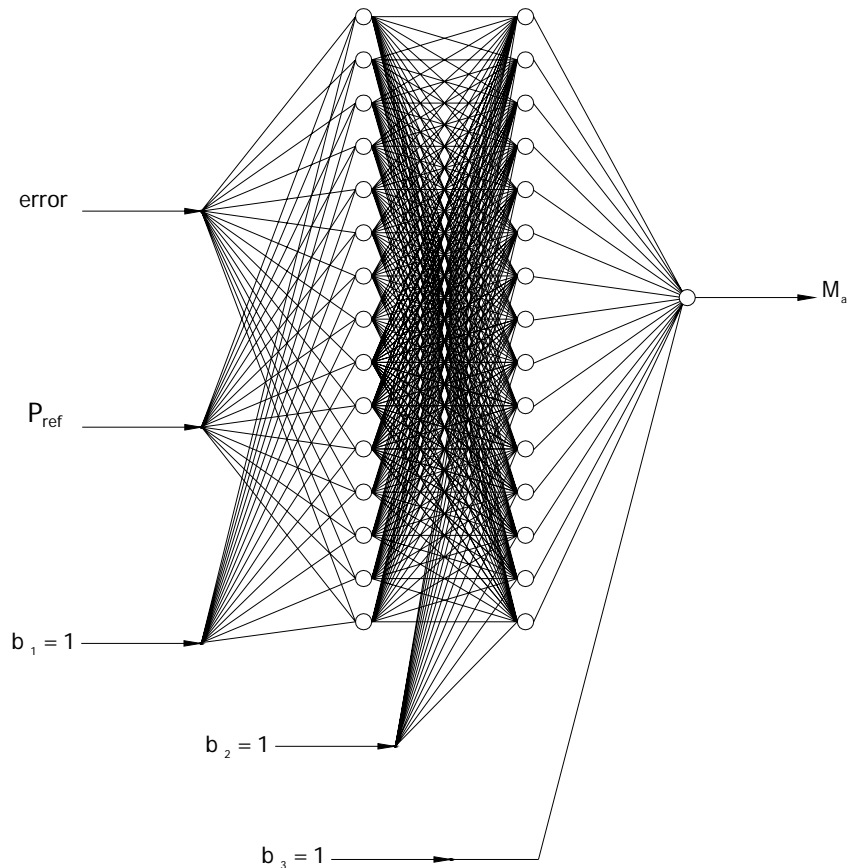
Figura 4.9: Red neuronal artificial con dos entradas dos capas ocultas de 15 neuronas cada una y una capa de salida con una sola neurona.
