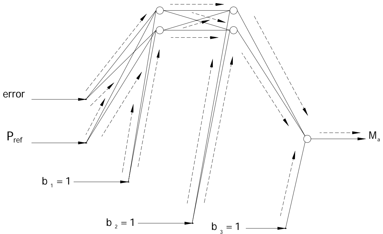
Figura 4.10: Propagación hacia delante de las señales de entrada desde los puntos de entrada, pasando por las capas ocultas, hasta la neurona de la capa de salida.
